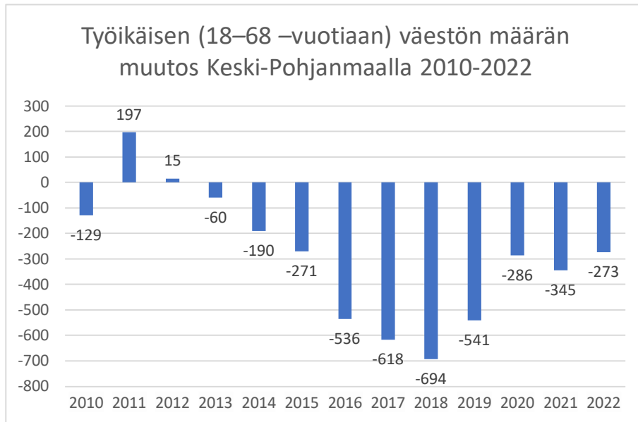
Kuva 4. Työikäisen (18–68-vuotiaan) väestön määrän muutos Keski-Pohjanmaalla vuosina 2010–2022. 6
