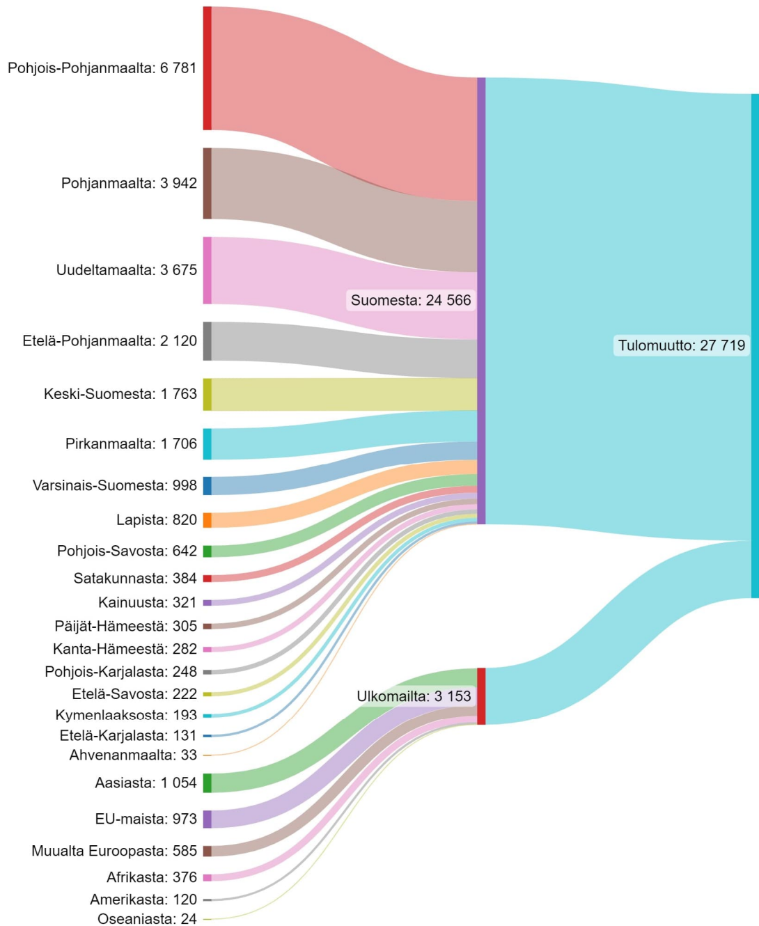
Kuva 2. Keski-Pohjanmaalle vuosina 2010–2022 muuttaneiden lähtöalueet. 4
