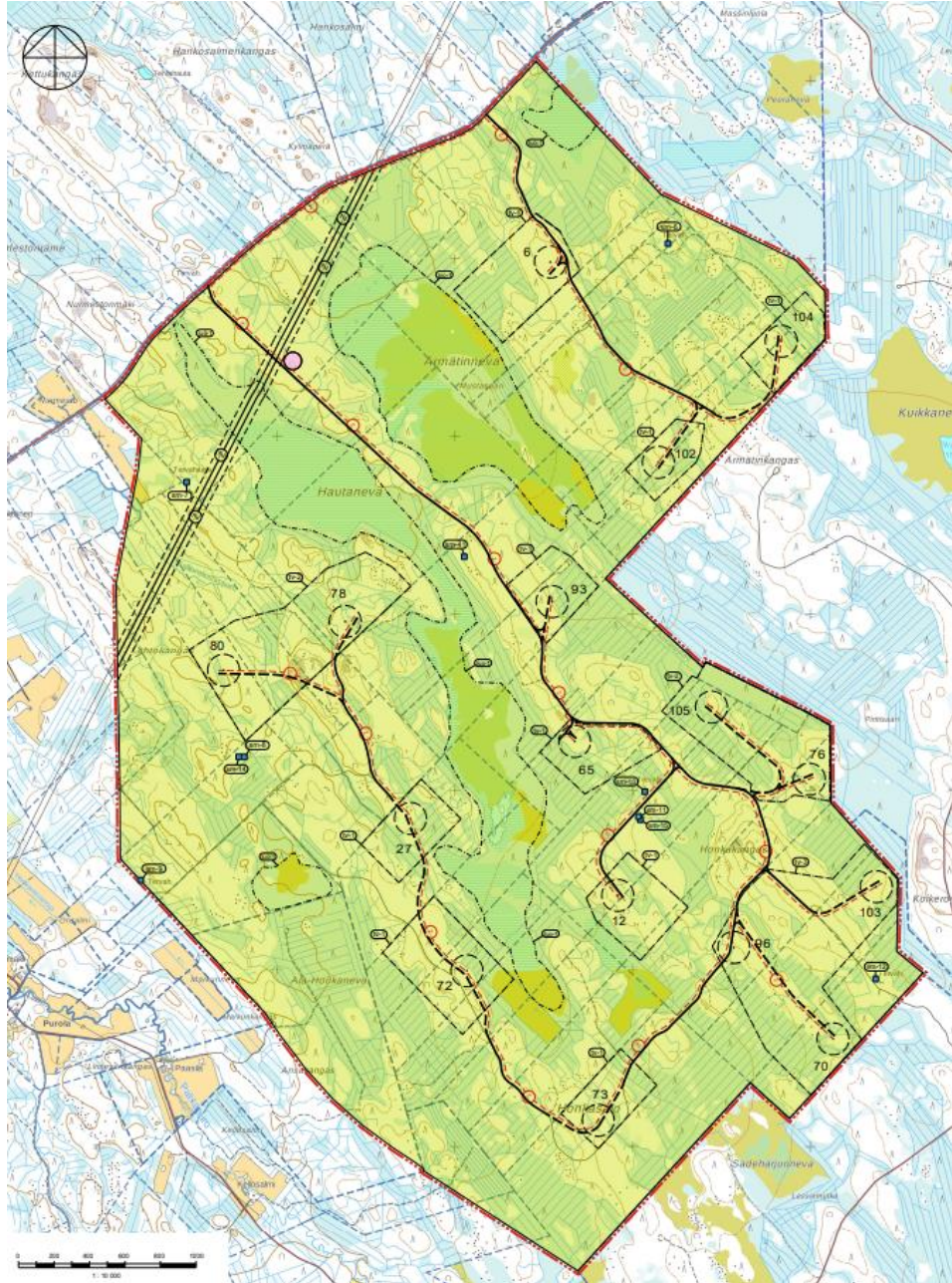
Osayleiskaavan mukainen voimalasijoittelu.
